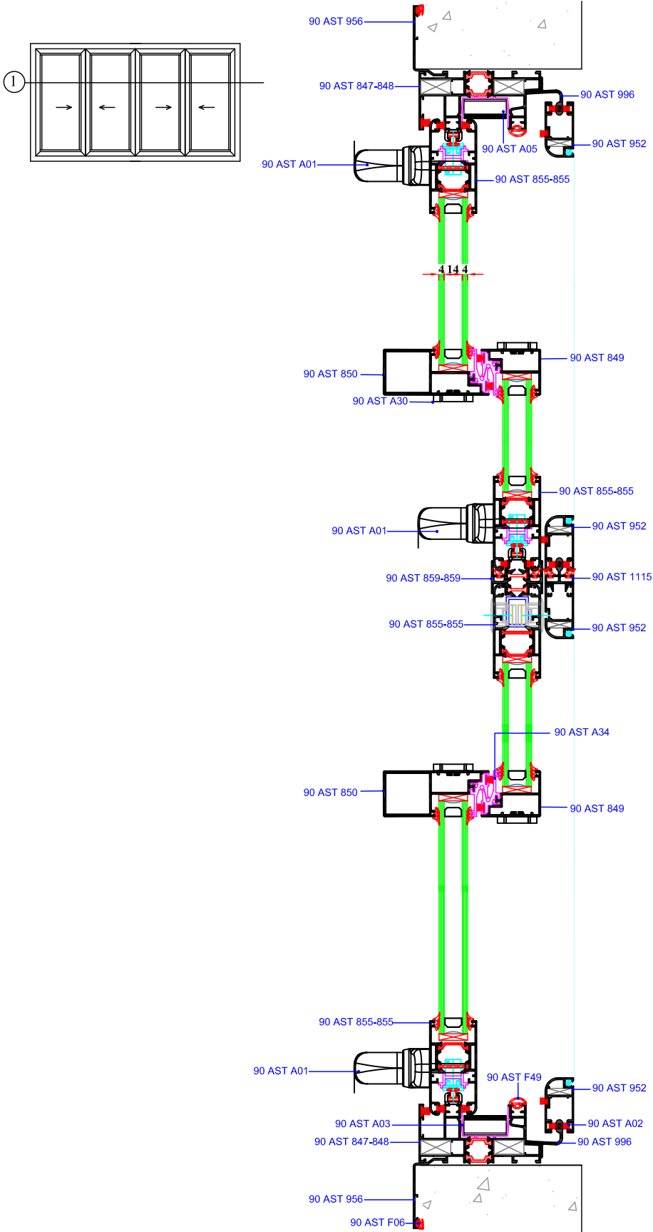
1 NOLU DETAY(4 KANATLI SÜRME )
