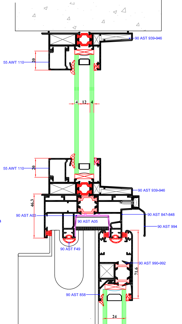
SABİT KANAT DETAYI
