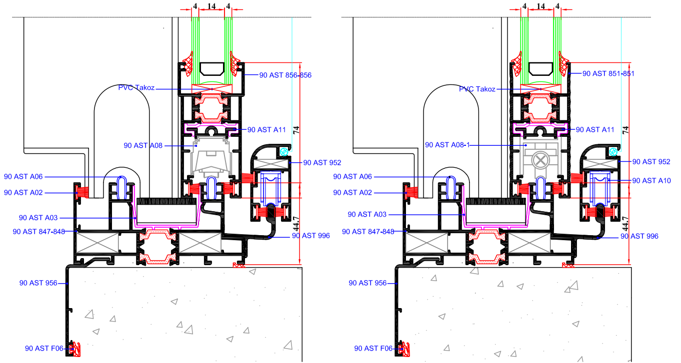
Teker Alternatif Detay
