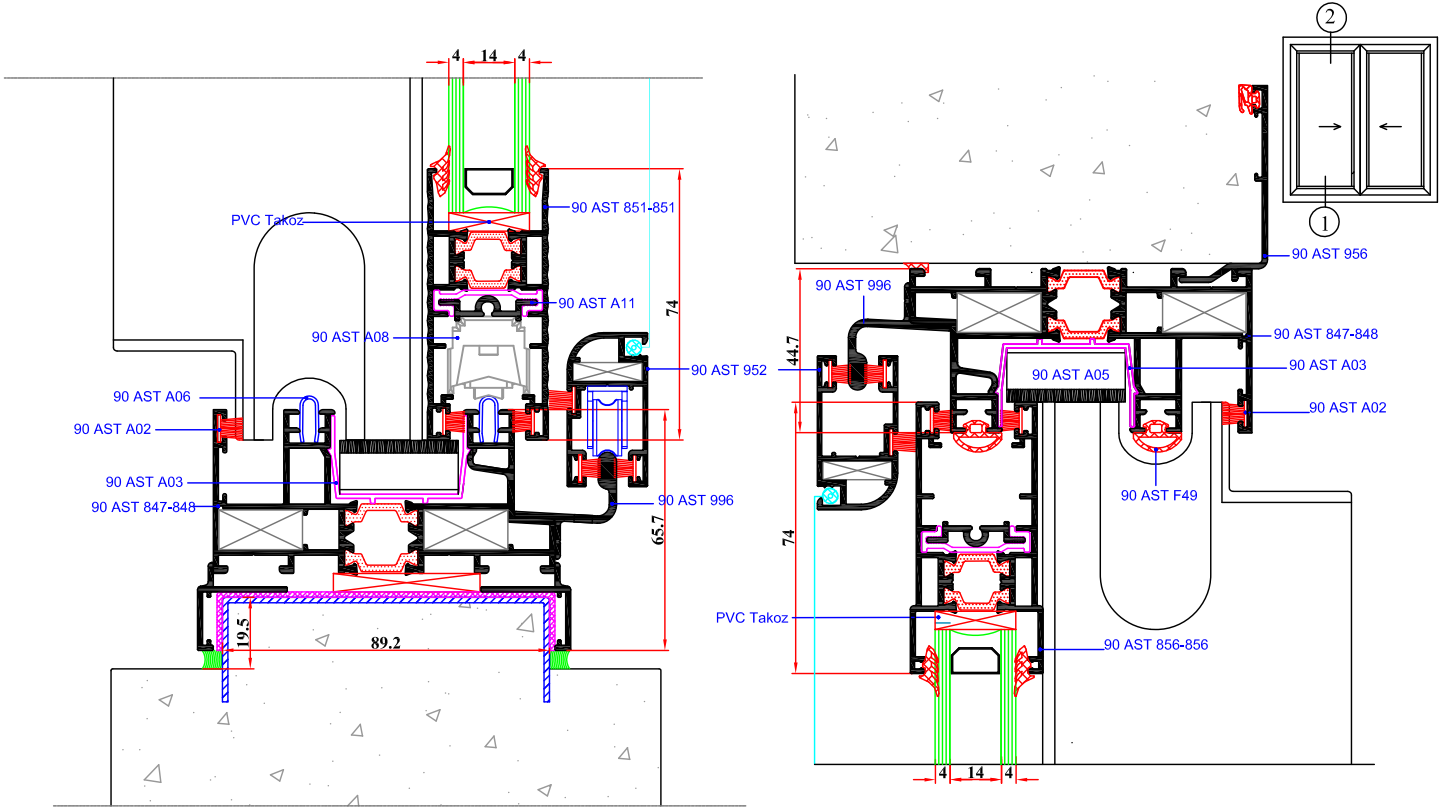
1 NOLU DETAY(Kör Kasalı Detay)
