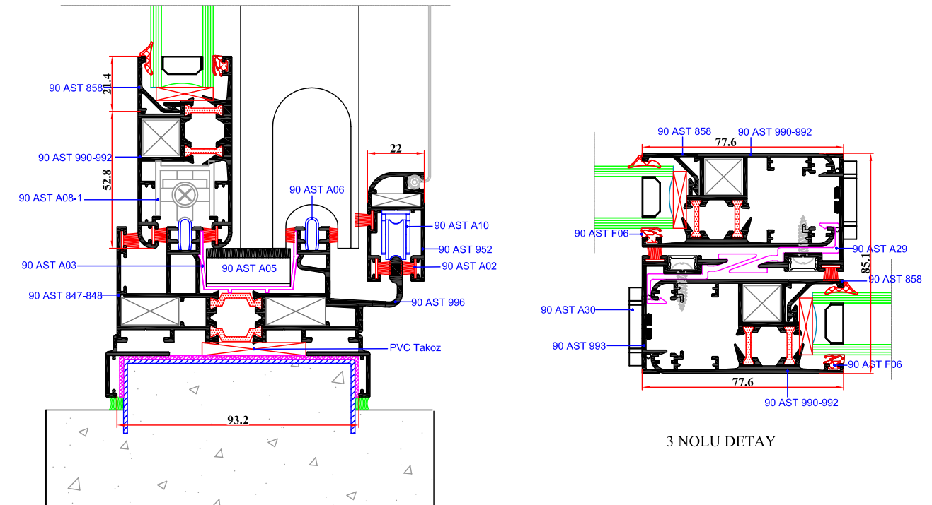
Teker Alternatif Detay
