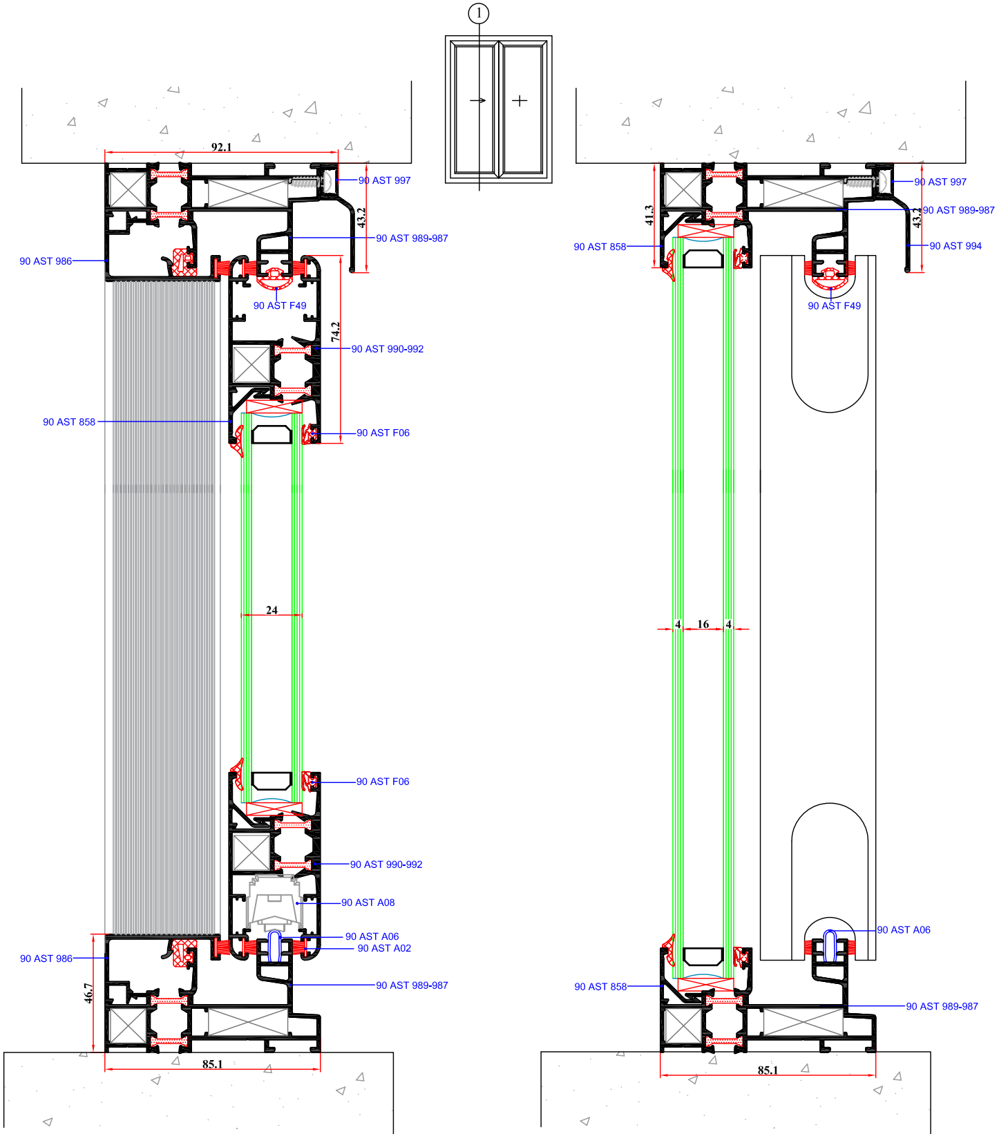
ÇITA ALTERNATİF DETAY
